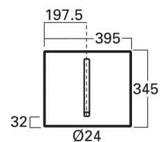
MINI HEADER
